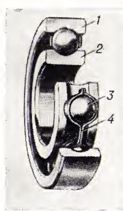
Рис. 1. Конструкция шарикоподшипника: 1 — наружное кольцо; 2 — внутреннее кольцо; 3 — шарик; 4 — сепаратор (штампованный).
